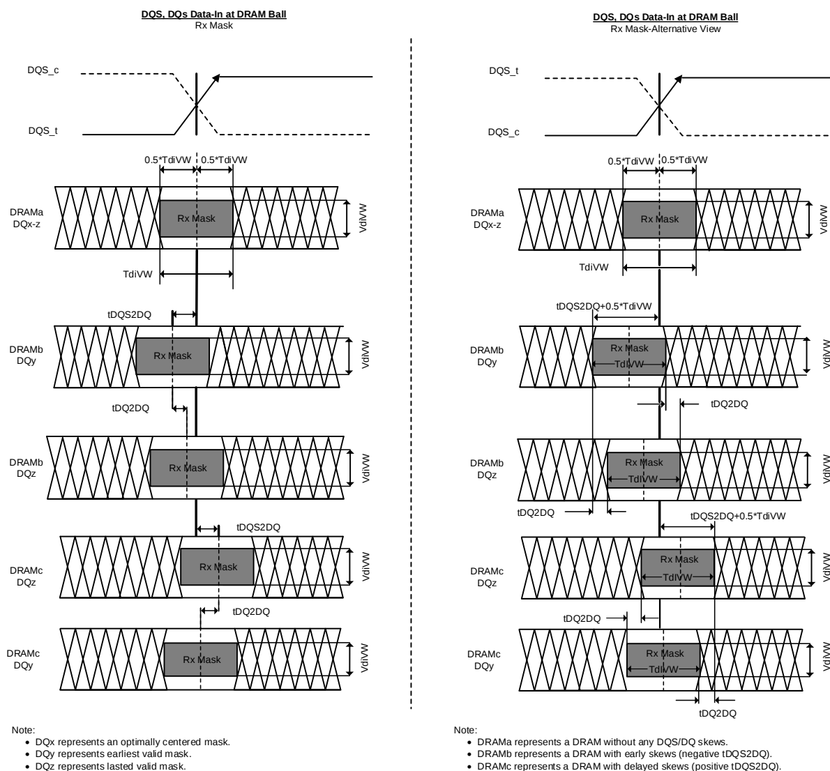
Figure 11-4. DQS to DQ and DQ to DQ Timings at DRAM Balls
